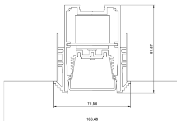
ГАБАРИТНЫЙ ЧЕРТЕЖ
