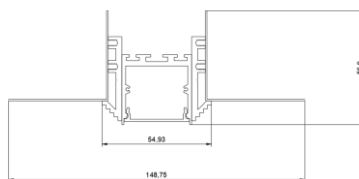
ГАБАРИТНЫЙ ЧЕРТЕЖ
