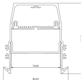
ГАБАРИТНЫЙ ЧЕРТЕЖ
