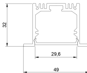
ГАБАРИТНЫЙ ЧЕРТЕЖ
