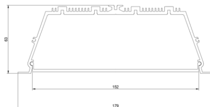
ГАБАРИТНЫЙ ЧЕРТЕЖ
