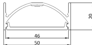
ГАБАРИТНЫЙ ЧЕРТЕЖ
