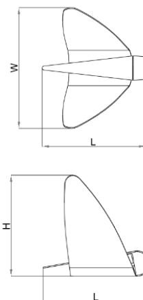
ГАБАРИТНЫЙ ЧЕРТЕЖ
