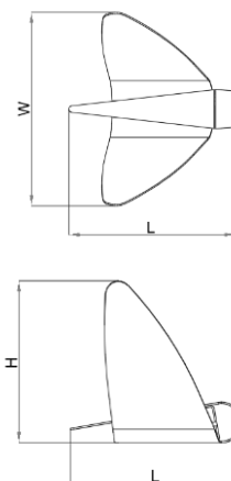
ГАБАРИТНЫЙ ЧЕРТЕЖ
