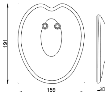
ГАБАРИТНЫЙ ЧЕРТЕЖ
