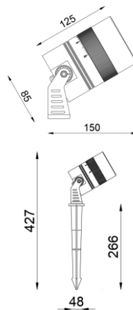
ГАБАРИТНЫЙ ЧЕРТЕЖ
