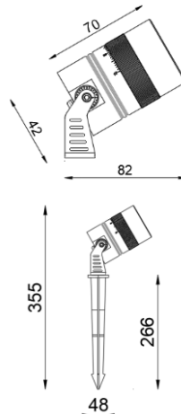
ГАБАРИТНЫЙ ЧЕРТЕЖ
