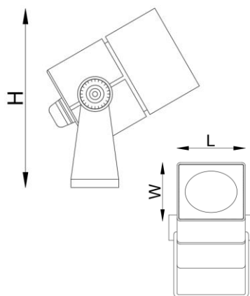
ГАБАРИТНЫЙ ЧЕРТЕЖ
