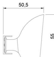
ГАБАРИТНЫЙ ЧЕРТЕЖ
