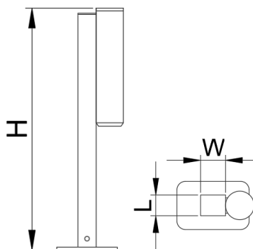
ГАБАРИТНЫЙ ЧЕРТЕЖ
