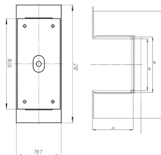
ГАБАРИТНЫЙ ЧЕРТЕЖ
