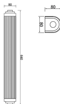
ГАБАРИТНЫЙ ЧЕРТЕЖ
