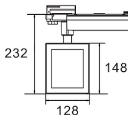
ГАБАРИТНЫЙ ЧЕРТЕЖ
