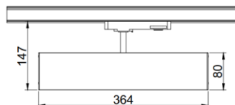
ГАБАРИТНЫЙ ЧЕРТЕЖ
