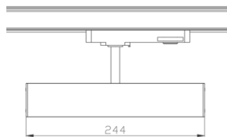
ГАБАРИТНЫЙ ЧЕРТЕЖ
