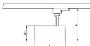
ГАБАРИТНЫЙ ЧЕРТЕЖ
