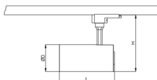
ГАБАРИТНЫЙ ЧЕРТЕЖ
