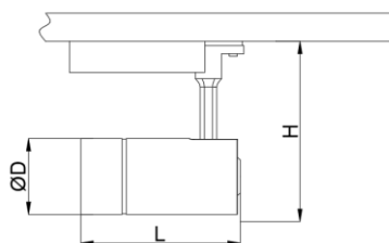
ГАБАРИТНЫЙ ЧЕРТЕЖ
