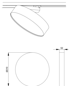
ГАБАРИТНЫЙ ЧЕРТЕЖ
