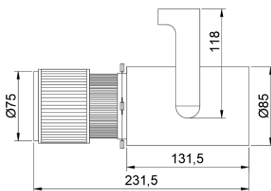
ГАБАРИТНЫЙ ЧЕРТЕЖ
