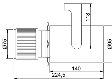
ГАБАРИТНЫЙ ЧЕРТЕЖ
