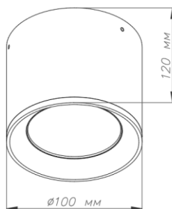
ГАБАРИТНЫЙ ЧЕРТЕЖ
