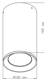
ГАБАРИТНЫЙ ЧЕРТЕЖ
