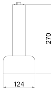
ГАБАРИТНЫЙ ЧЕРТЕЖ
