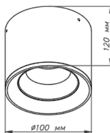
ГАБАРИТНЫЙ ЧЕРТЕЖ
