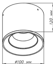
ГАБАРИТНЫЙ ЧЕРТЕЖ
