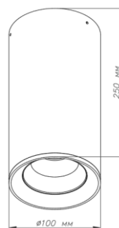
ГАБАРИТНЫЙ ЧЕРТЕЖ
