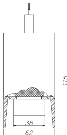
ГАБАРИТНЫЙ ЧЕРТЕЖ
