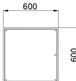
ГАБАРИТНЫЙ ЧЕРТЕЖ
