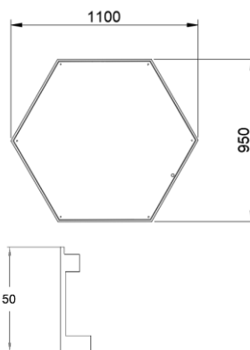
ГАБАРИТНЫЙ ЧЕРТЕЖ
