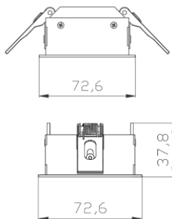
ГАБАРИТНЫЙ ЧЕРТЕЖ
