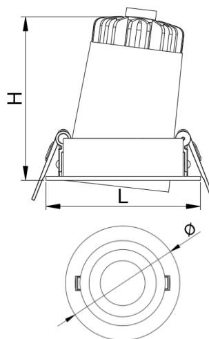
ГАБАРИТНЫЙ ЧЕРТЕЖ
