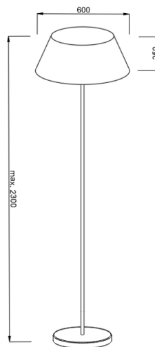
ГАБАРИТНЫЙ ЧЕРТЕЖ
