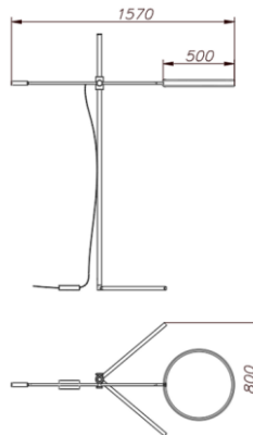
ГАБАРИТНЫЙ ЧЕРТЕЖ
