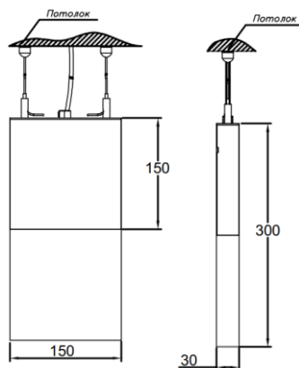
ГАБАРИТНЫЙ ЧЕРТЕЖ
