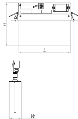
ГАБАРИТНЫЙ ЧЕРТЕЖ
