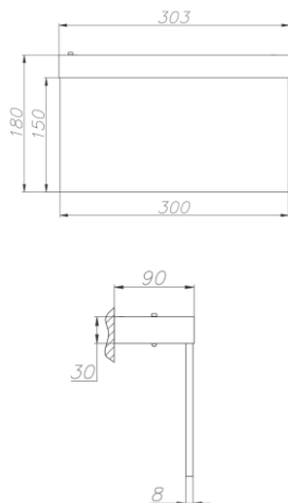
ГАБАРИТНЫЙ ЧЕРТЕЖ
