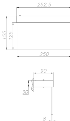
ГАБАРИТНЫЙ ЧЕРТЕЖ
