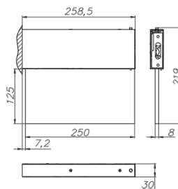
ГАБАРИТНЫЙ ЧЕРТЕЖ
