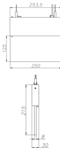
ГАБАРИТНЫЙ ЧЕРТЕЖ
